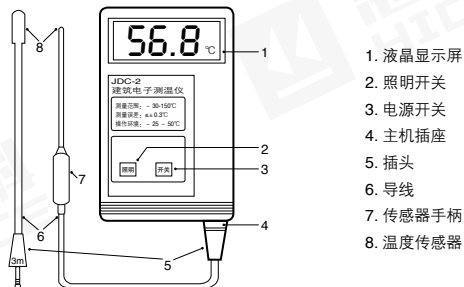
测温仪主机、测温探头和测温线示意图
